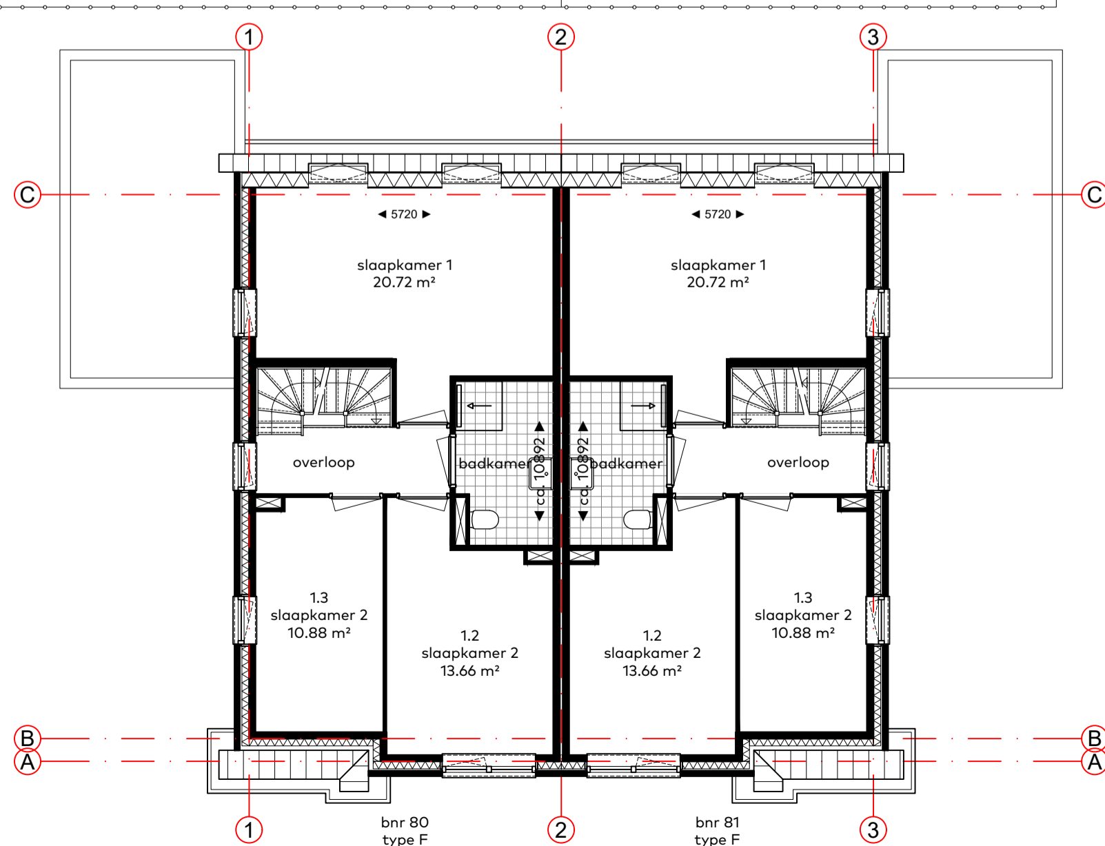
VERDIEPING bnr 80 type F bnr 81 type F
