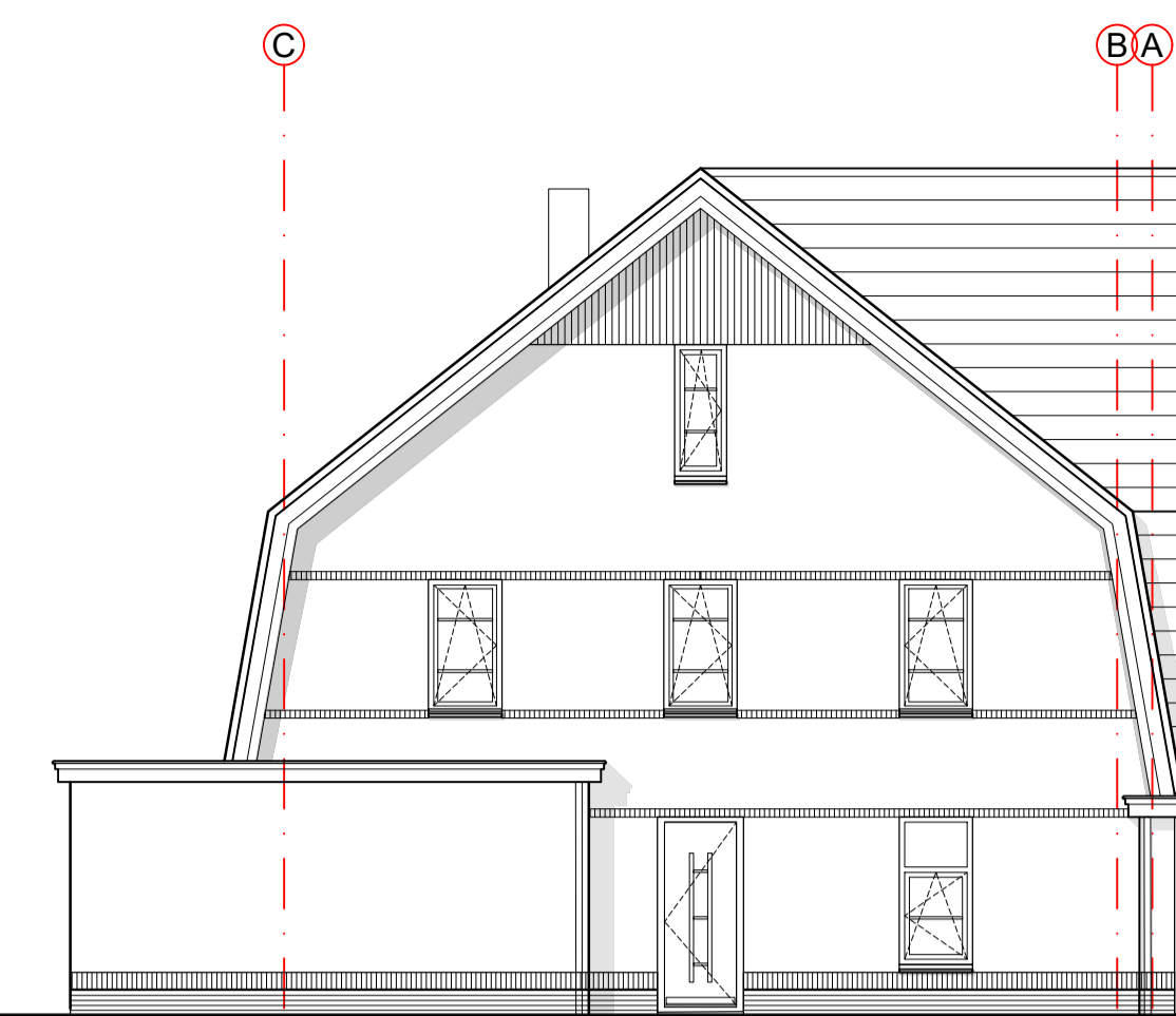
LINKER ZIJGEVEL bnr 80 type F
