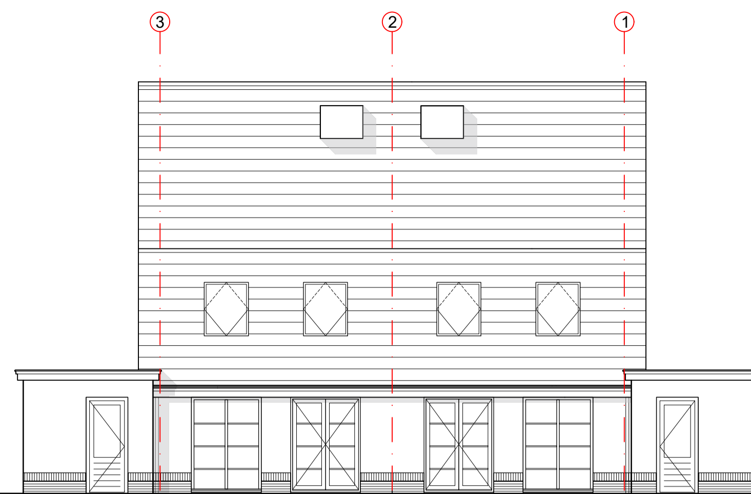
ACHTERGEVEL bnr 81 type F bnr 80 type F
