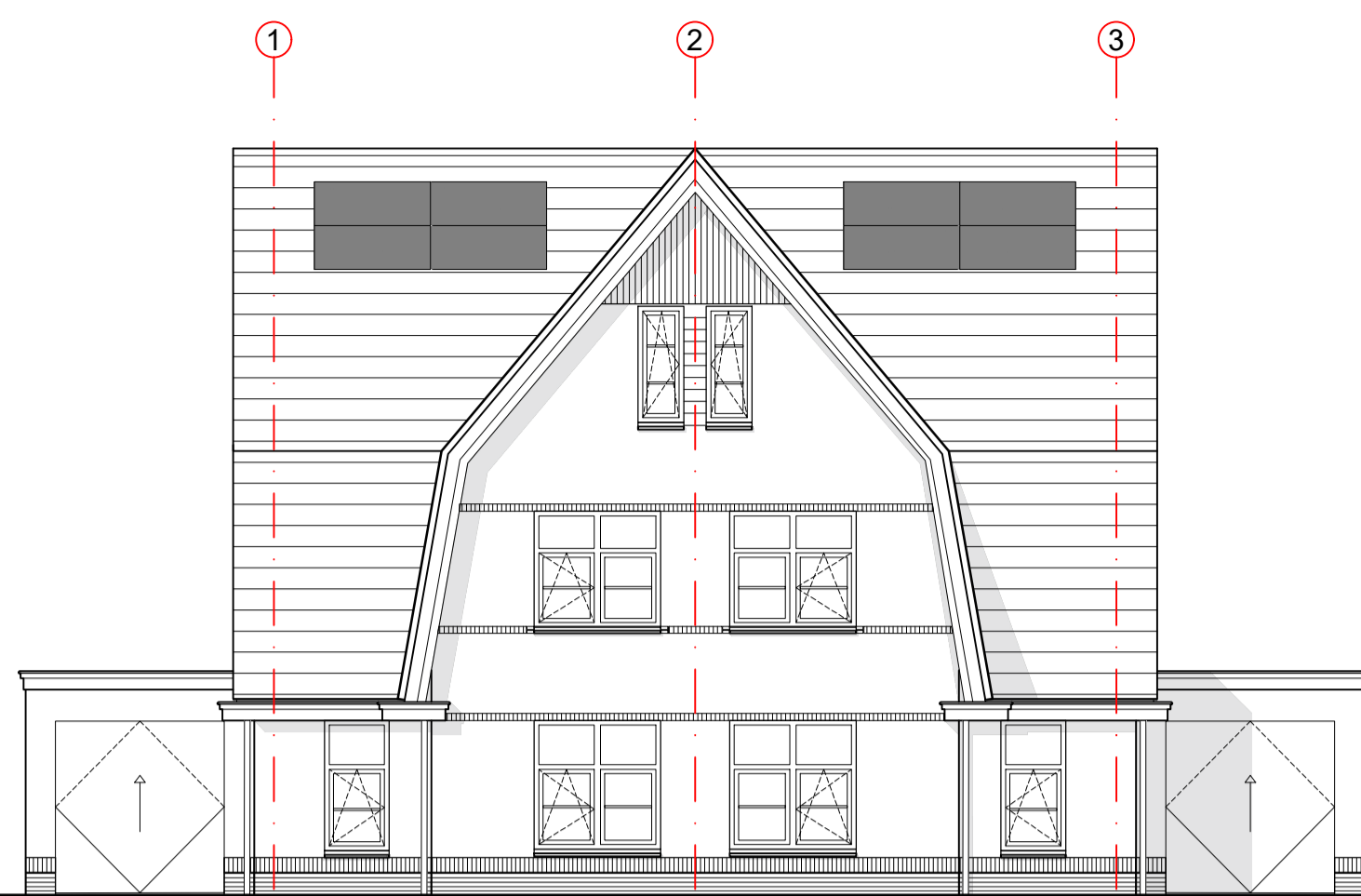
VOORGEVEL bnr 80 type F bnr 81 type F
