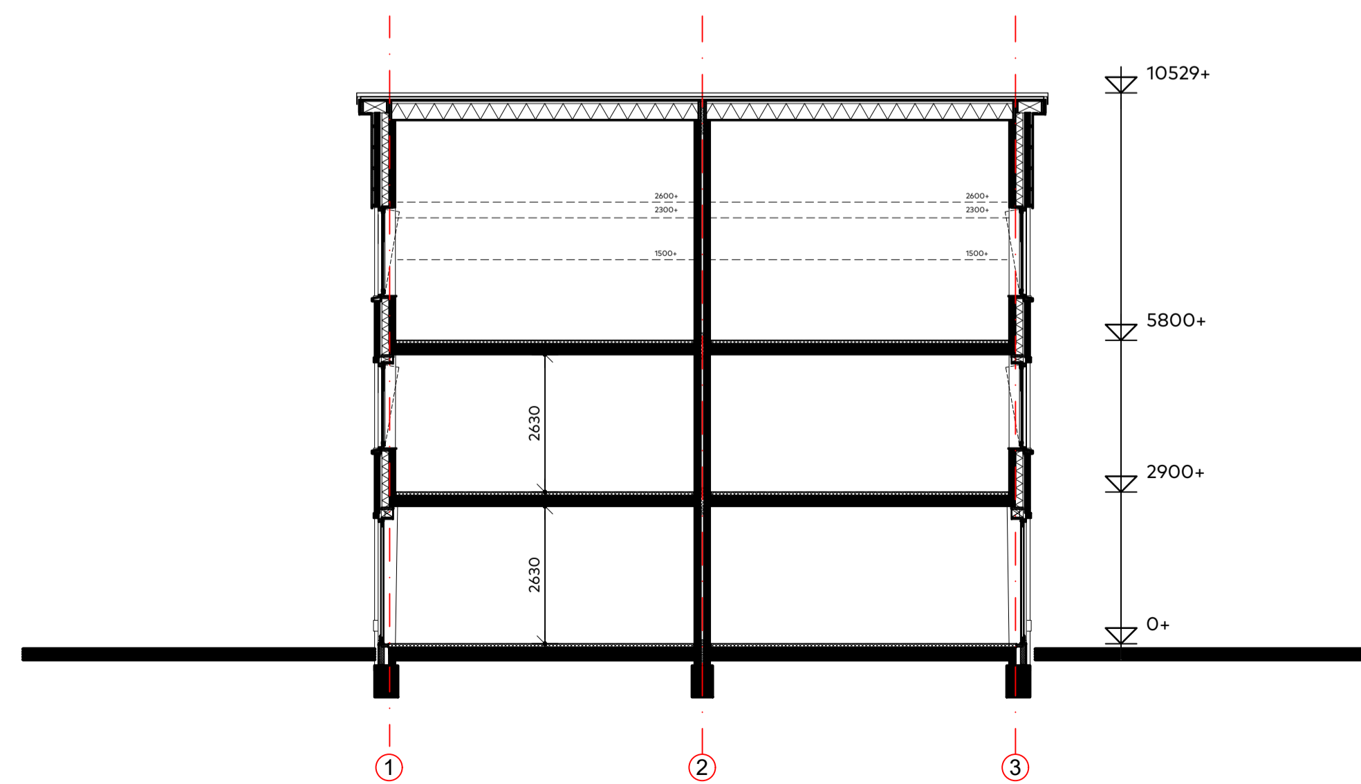
principe doorsnede type F
