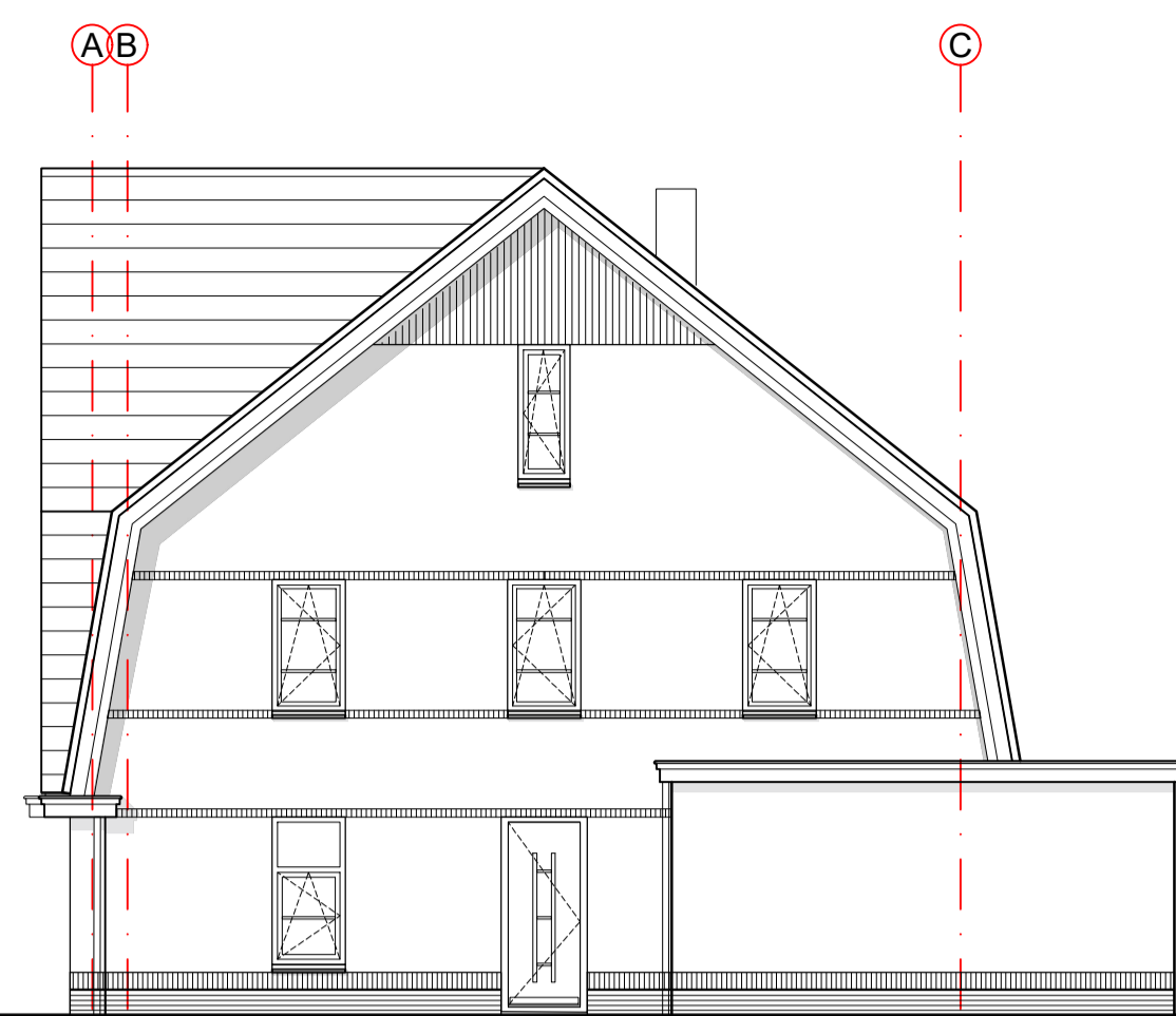
RECHTER ZIJGEVEL bnr 81 type F
